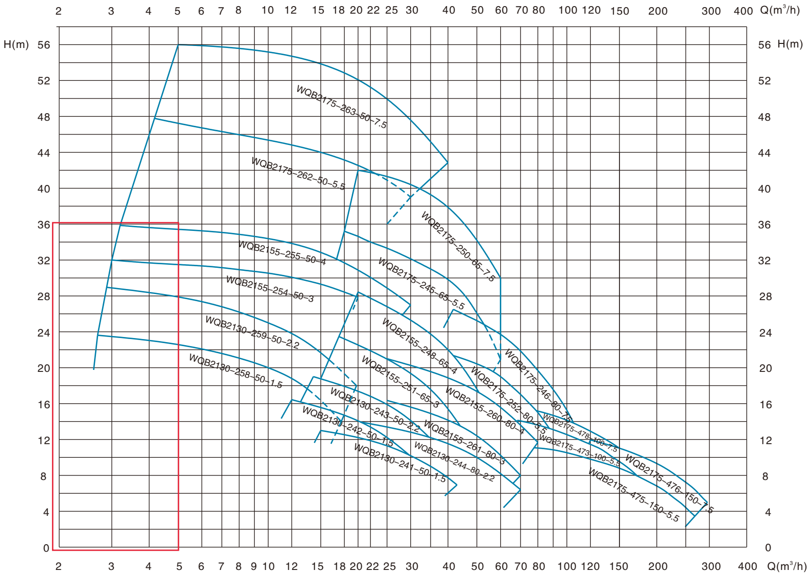
WQB防爆型潜水排污泵型谱图
