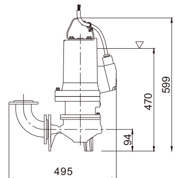
Y 硬管移动式安装
