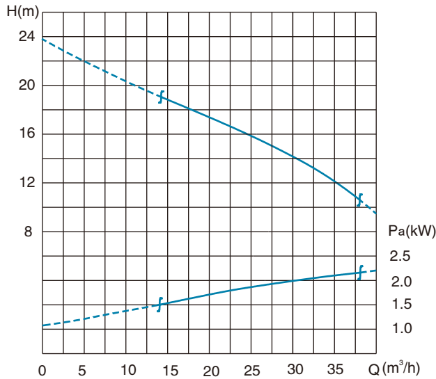
性能曲线图
