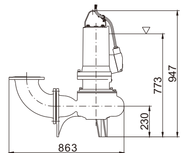
Y 硬管移动式安装
