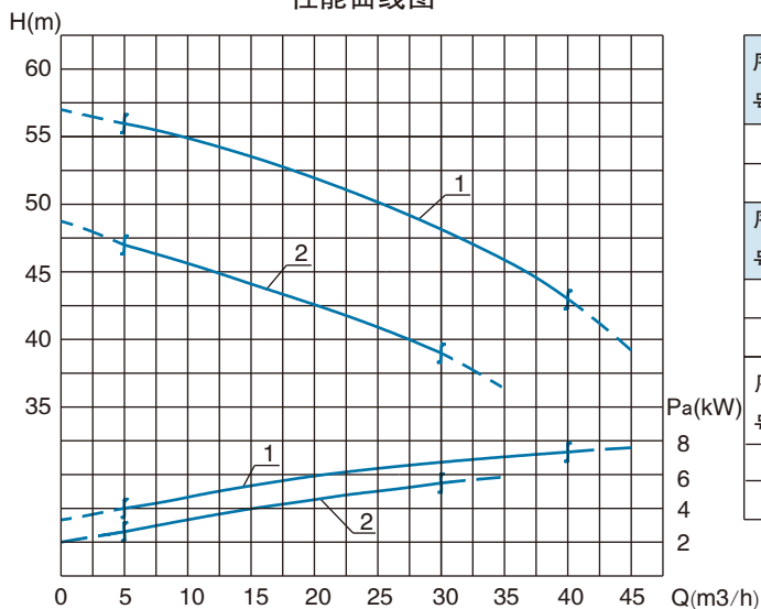
性能曲线图
