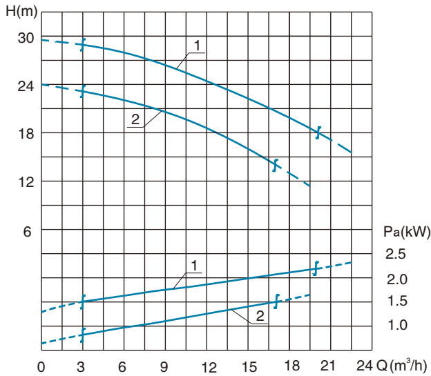
性能曲线图
