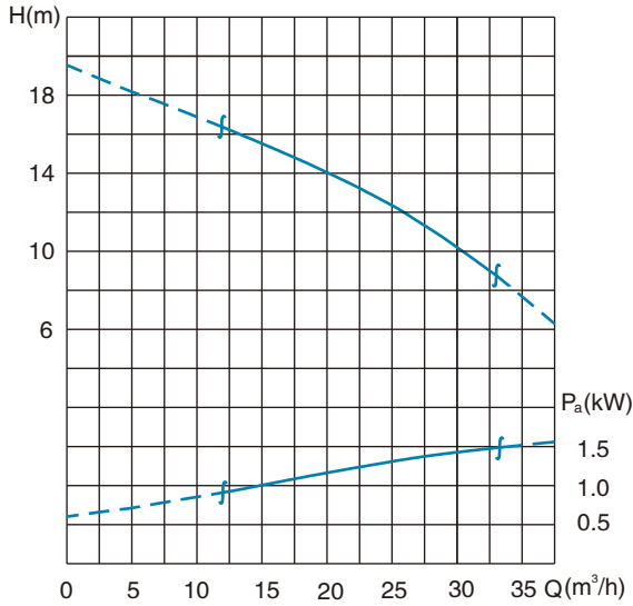
性能曲线图
