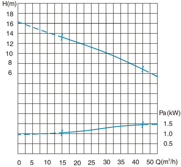
性能曲线图
