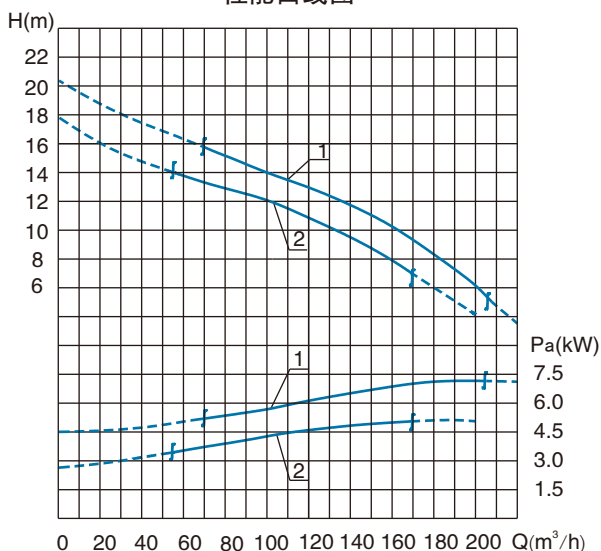
性能曲线图
