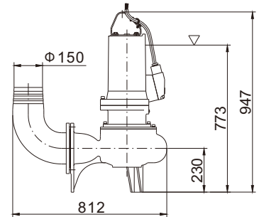
R 软管移动式安装
