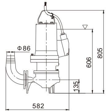
R 软管移动式安装
