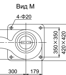
Монтаж на кольцевом основании (P)
