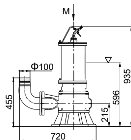
Монтаж в переносном варианте со шлангом (R)
