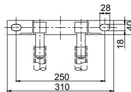
Вид В
