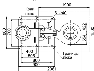
Вид А
