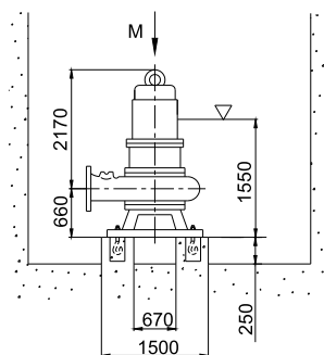
Монтаж на кольцевом основании (P)
