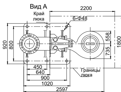
Монтаж на кольцевом основании (P)
