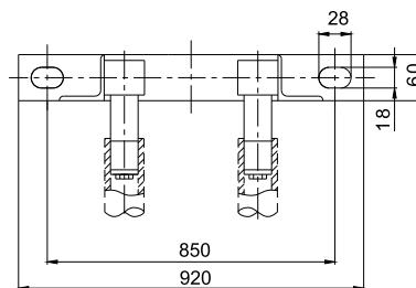
Вид В
