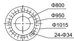
Размер фланца
