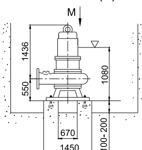
Монтаж на кольцевом основании (P)
