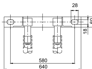
Вид В
